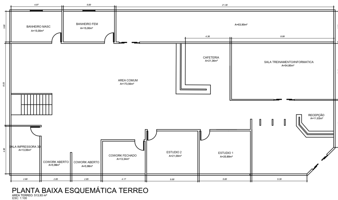
Figura 4 — Planta Baixa do Centro de Empreendedorismo e Inovação
